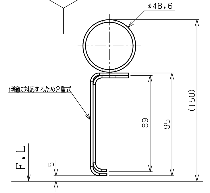
A-巾木部詳細図 S=1/2
