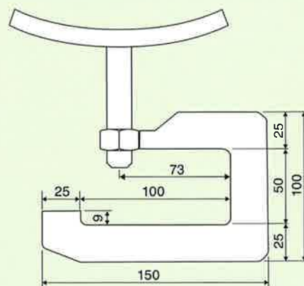
プレート寸法概略
